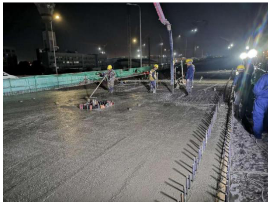
图2 混凝土浇筑
