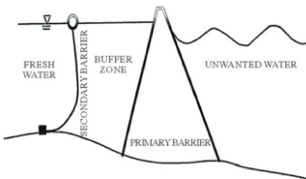
Figure 4: Soft dam concept, Yang et al, 2005 [2]
